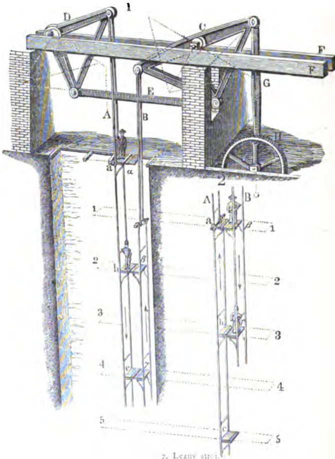
7. Lezný stroj.
